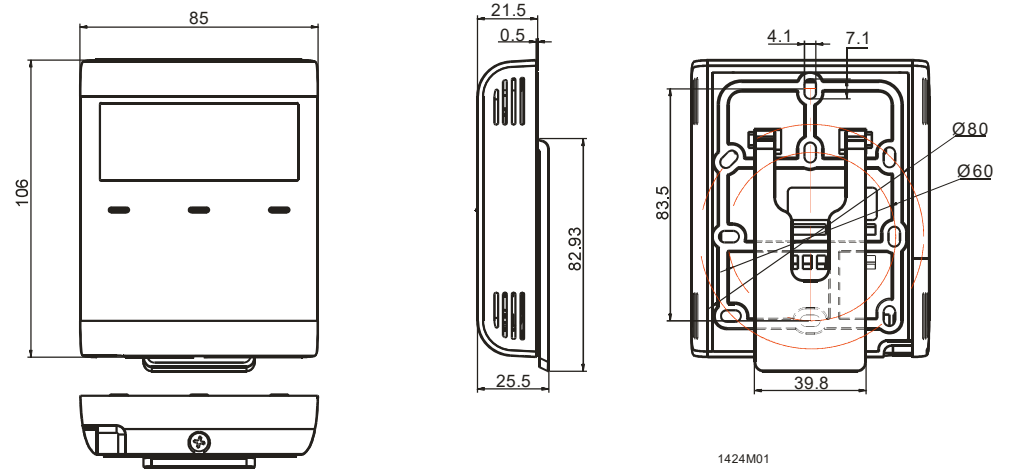
Prostorový regulátor RDD100.1RF
