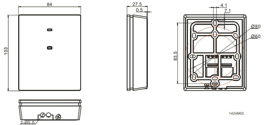
Přijímač RCR100RF
