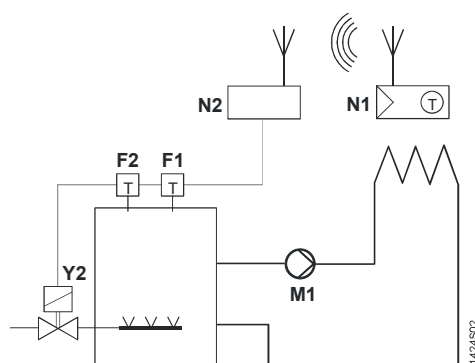
Bezdrátový regulátor a spínací jednotka regulují prostorovou teplotu přímým řízením závěsného plynového kotle.
